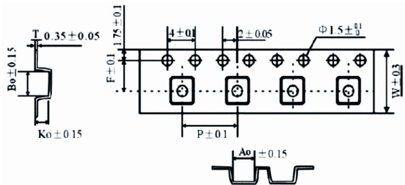
编带尺寸 Dimensions of tape(unit:mm)
